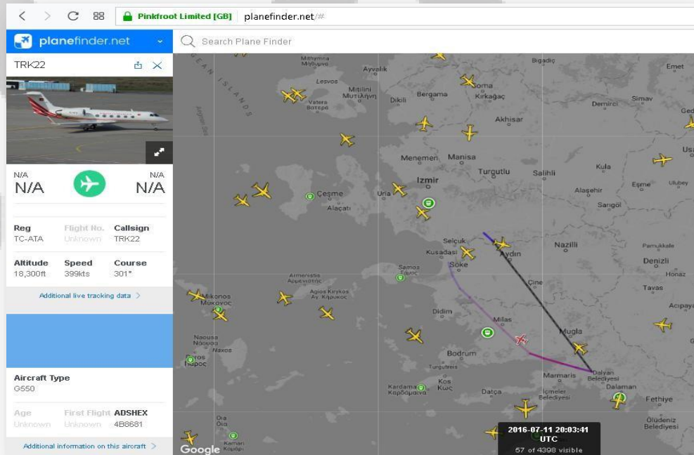
Şekil 7 TC-ATA Dalaman-A.Menderes 22.55-23.20
