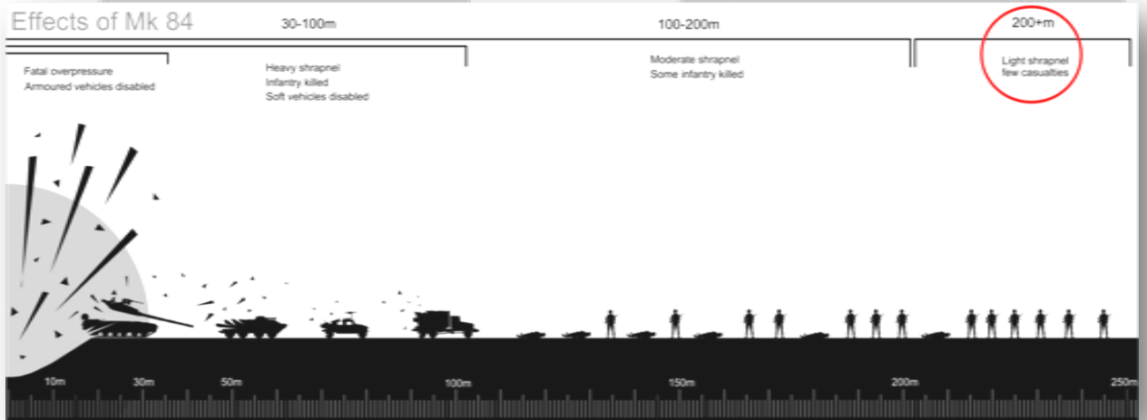
Şekil 26 MK-84 bombasının parça tesir mesafesinde verdiği zarar
