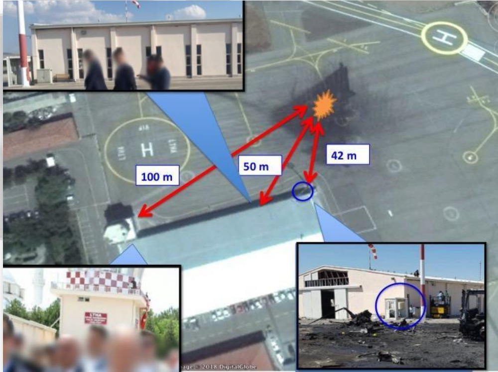
Şekil 48 Helikopter Pistine atılan bombadan etkilenen bölgeler ve mesafeler
